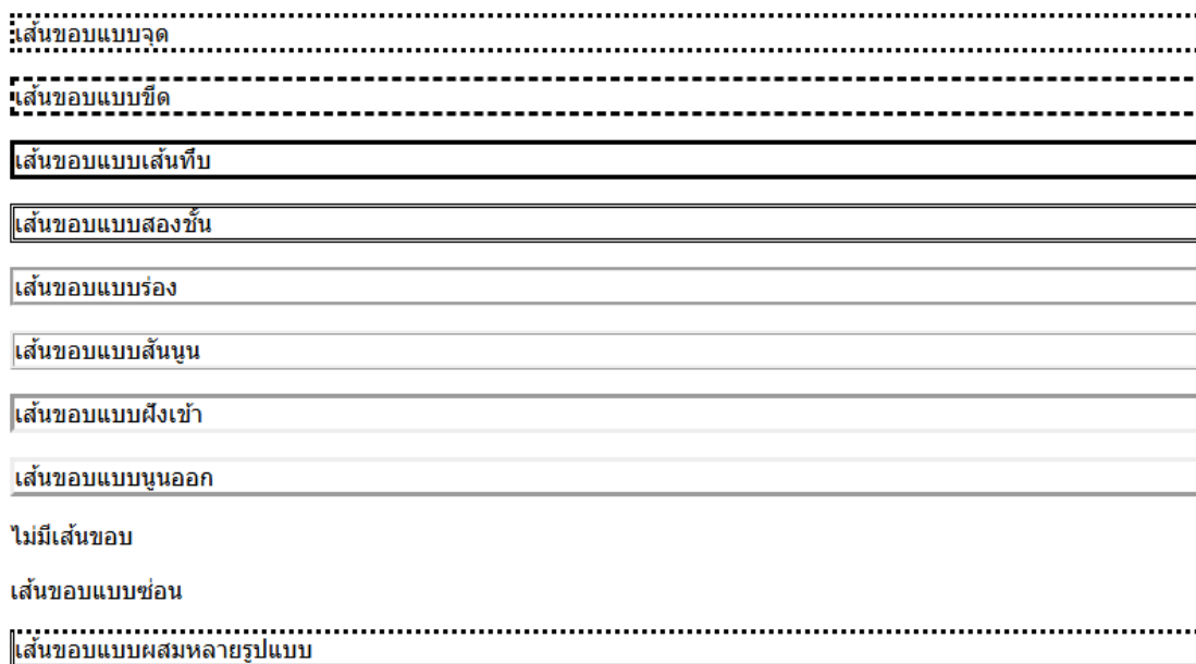
ภาพที่ 2.2 ตัวอย่างรูปแบบ Border ใน CSS
