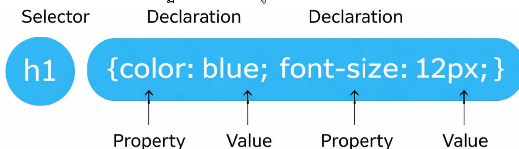
ภาพที่ 2.1 โครงสร้างการเรียกใช้ CSS ให้กับ element ของ html
